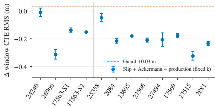
(d) Paired CTE difference, mean and 95% CI
