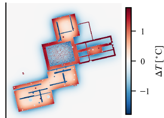
(d) high-pass residual T - G_{\sigma}(T) (defect enhancement)
