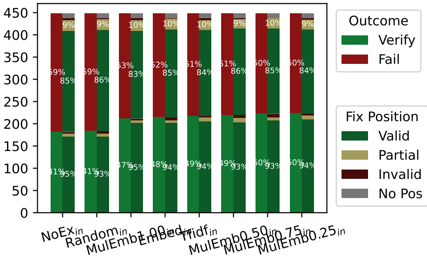
Testcases
