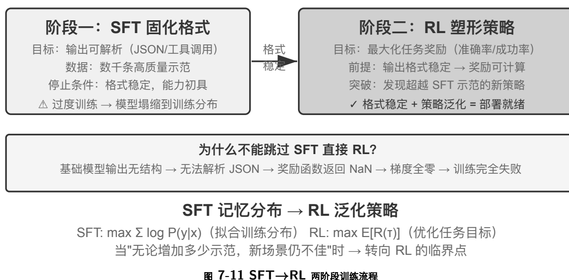
图 7-11 SFT→RL 两阶段训练流程
