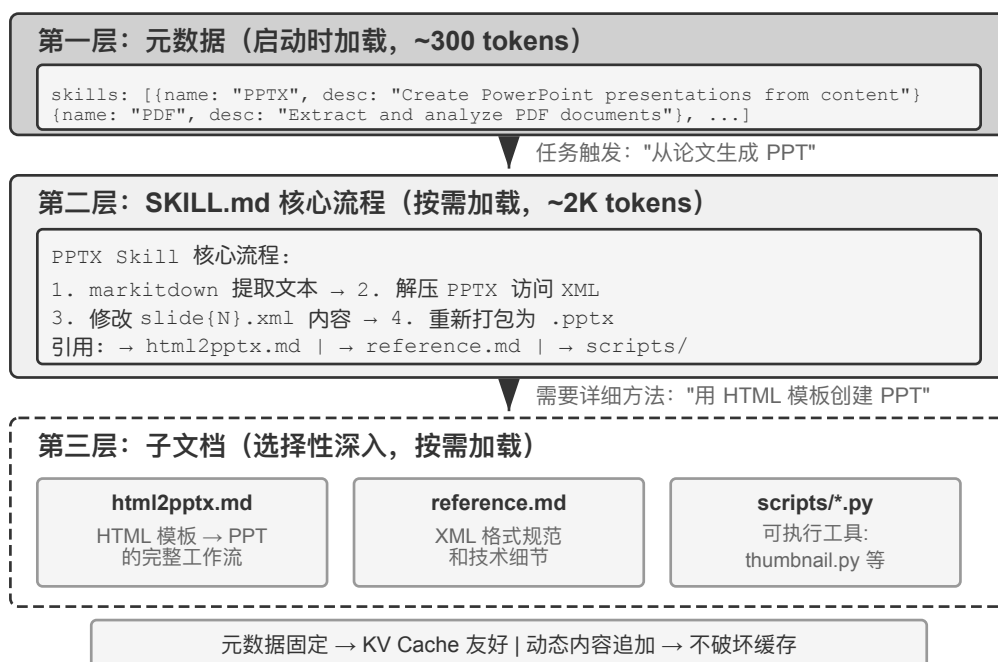
图 2-11 Skills 渐进式披露机制
