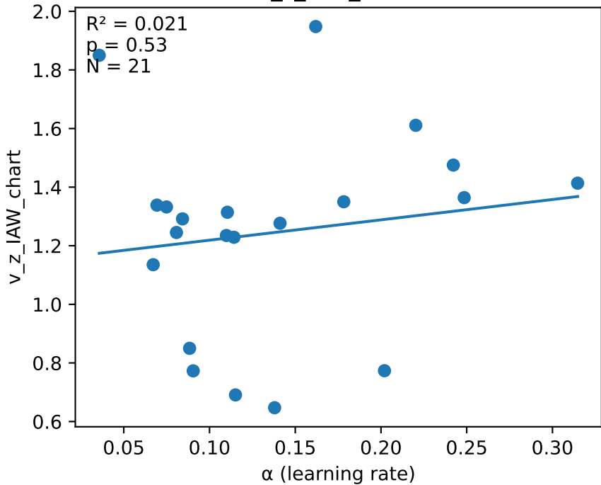
v_z_IAW_chart
