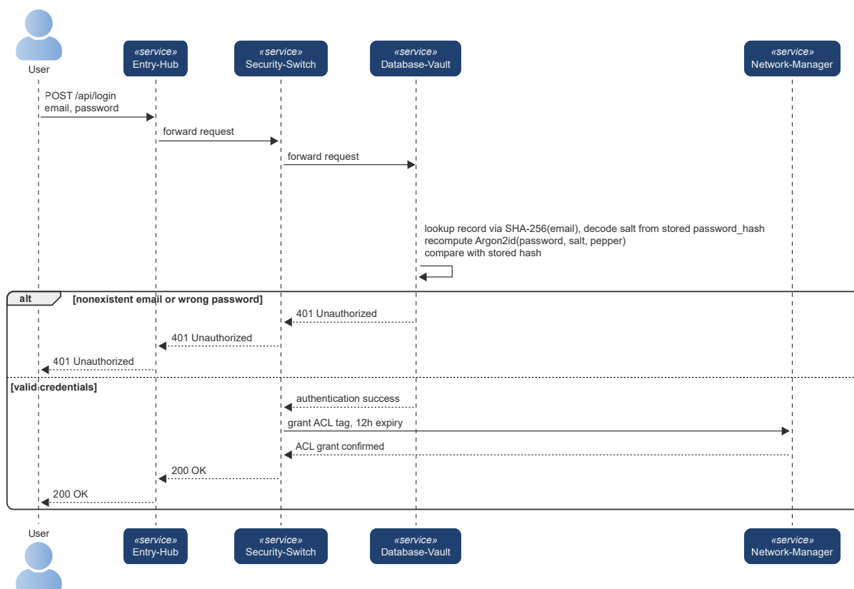
Figura 5.2: Sequenza di autenticazione (UC-02).
