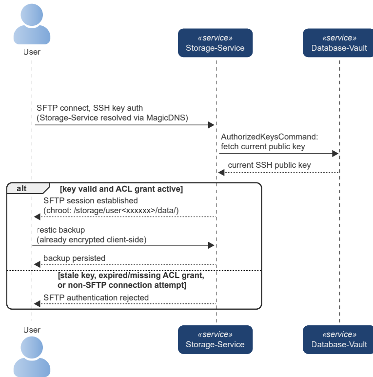
Figura 6.1: Sequenza di backup di un file (UC-03).
