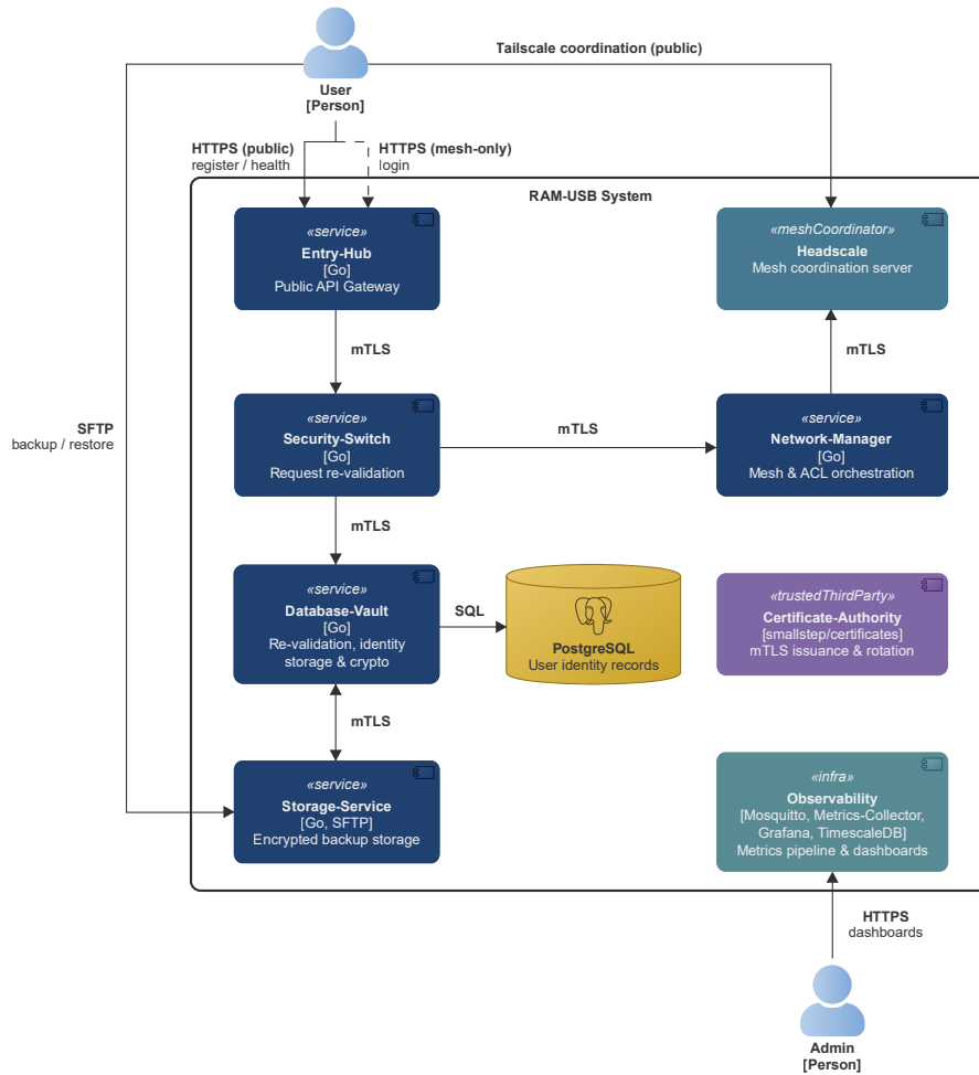
Figura 4.3: Diagramma dei container di RAM-USB.
