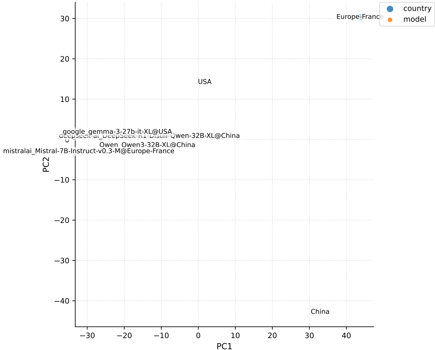
Mapa de proximidad (PCA 2D) - Var exp: PC1=0.53, PC2=0.34
