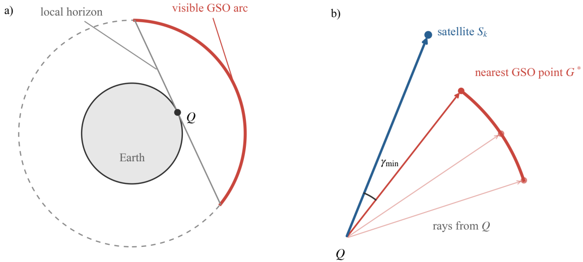
Рис. 6: Схема геозащитной маски для произвольной точки Q (не в масштабе): а) локальный горизонт выделяет видимую дугу ГСО; б) каждый красный луч соединяет Q с одной из точек G(\ell) этой дуги. Точка G^* выбирается так, чтобы угол между лучами на G^* и на КА S_k был минимальным.
