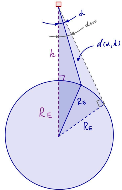
Рис. 7: Геометрия задачи: высота спутника h , наклонная дальность d_{\max} и максимальный угол обзора \alpha_{\max} .
