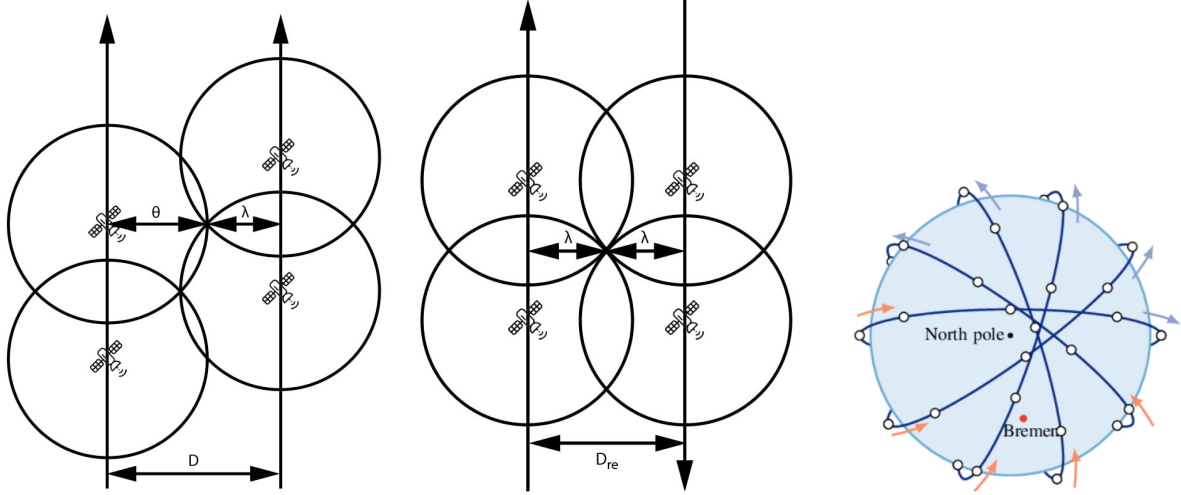
(а) Коорбитальные условия: соседние плоскости движутся в одном направлении; показаны полоса покрытия и фазовый сдвиг. (б) Ретроградные условия: соседние плоскости движутся в противоположных направлениях; показан суммарный эффект полос покрытия. (с) Полярные условия: иллюстрация области вокруг полюса и требование перекрытия "слабообласти" для обеспечения покрытия.
