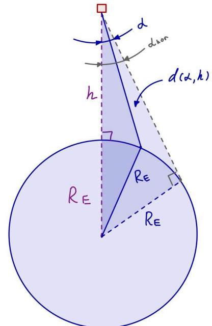
Рис. 8: Геометрия задачи: высота спутника h , наклонная даль-
