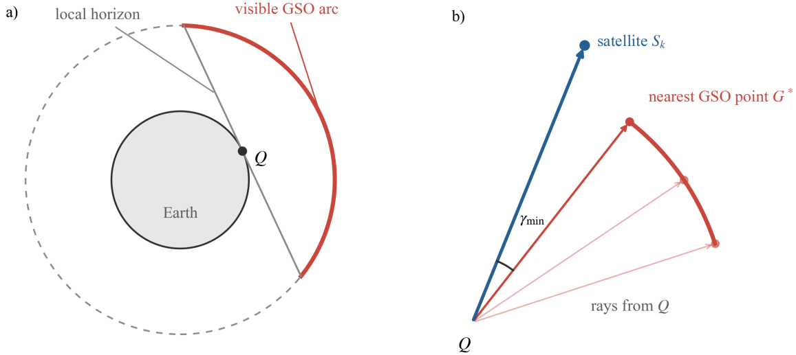
Рис. 7: Схема геозащитной маски для произвольной точки Q (не в масштабе): а) локальный горизонт выделяет видимую дугу ГСО; б) каждый красный луч соединяет Q с одной из точек G(\ell) этой дуги. Точка G^* выбирается так, чтобы угол между лучами на G^* и на КА S_k был минимальным.
