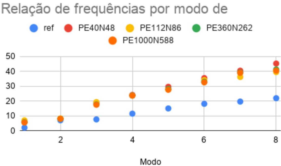
Figura 5.24 – Relação de frequências por modo de vibração para a parede estrutural.
