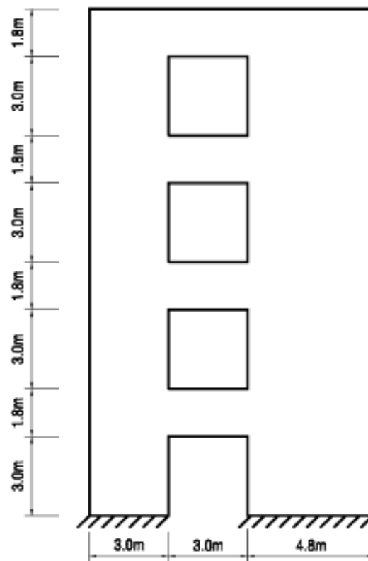
Figura 5.22 – Geometria e modelo da parede estrutural.
