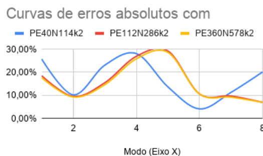
Figura 5.28 – Curvas de erros absolutos com o parâmetro de estabilização de: a) Park et al. e b) Antonietti et al.
