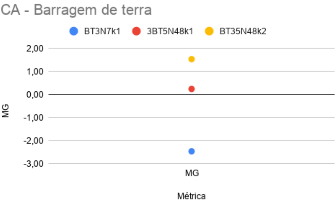
Figura 5.21 – Coeficiente de acurácia relativo da barragem de terra.
