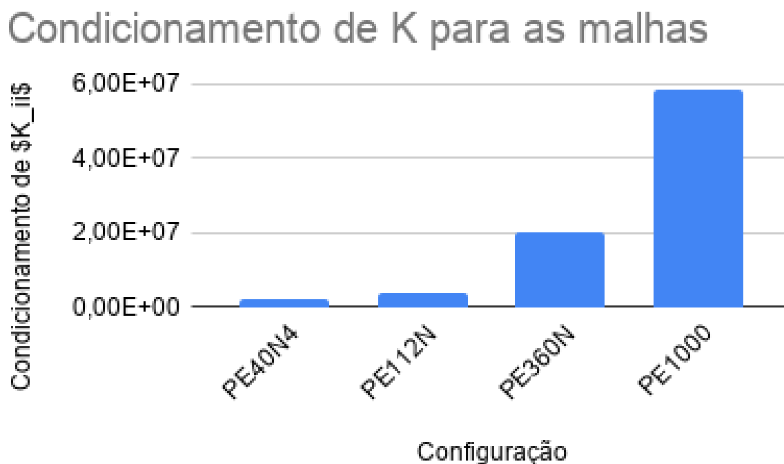
Figura 5.25 – Condicionamento da matriz K para as malhas triangulares de primeira ordem.
