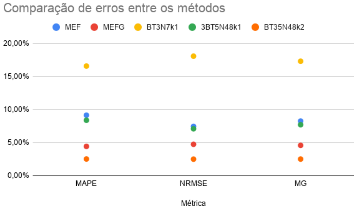
Figura 5.20 – Comparação de erros entre os métodos numéricos.
