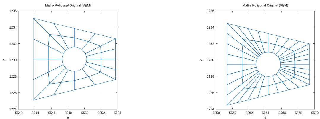
Figura 5.3 – Malhas de 32 e 64 elementos
