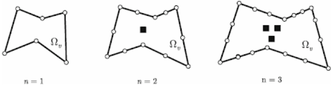
Figura 4.5 – Geometria do elemento.
