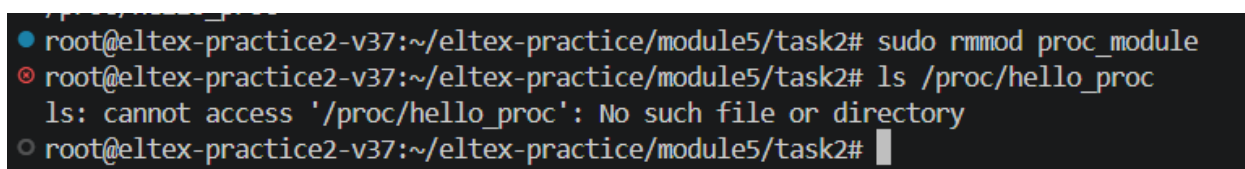
Рисунок 6 – Удаление модуля
