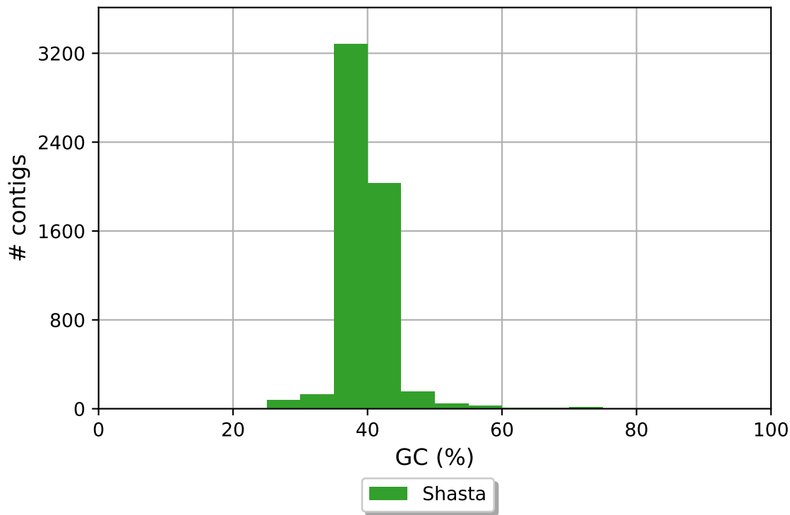
Shasta GC content
