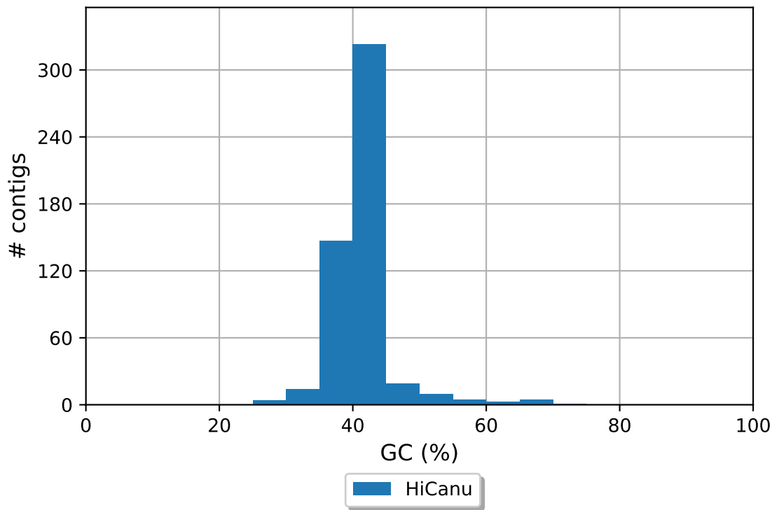
HiCanu GC content
