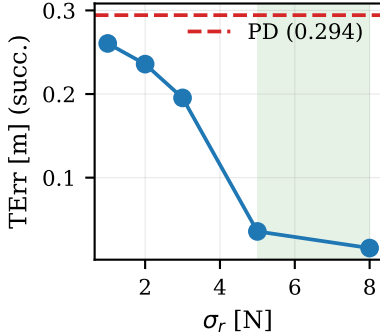
(b) Terminal error
