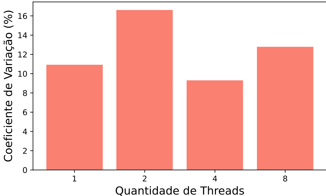
K-Means Coef. de Variação por Tempo de Exec.
