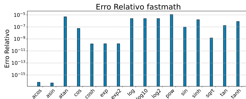
Figura 6 – Erro relativo entre as funções da fastmath .
