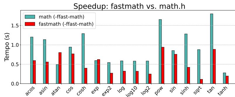
Figura 5 – Comparativo de speedup entre a biblioteca fastmath e a math .
