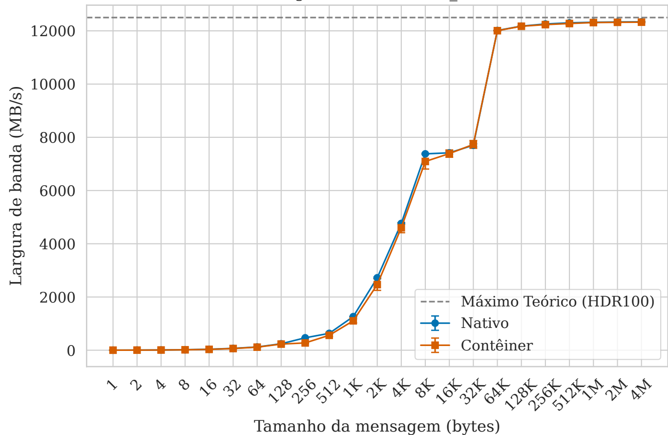
Largura de Banda (osu_bw)
