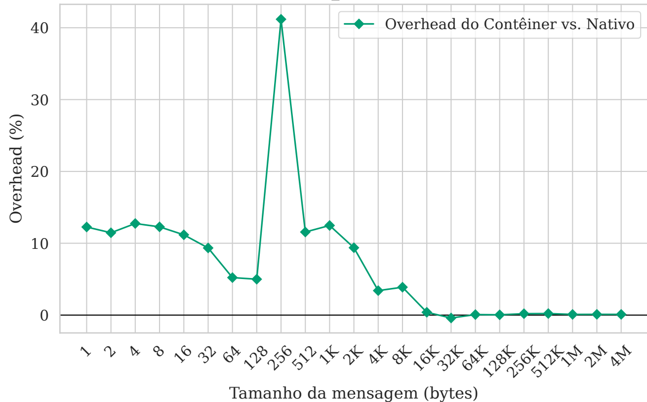
Largura de Banda (osu_bw): overhead do contêiner
