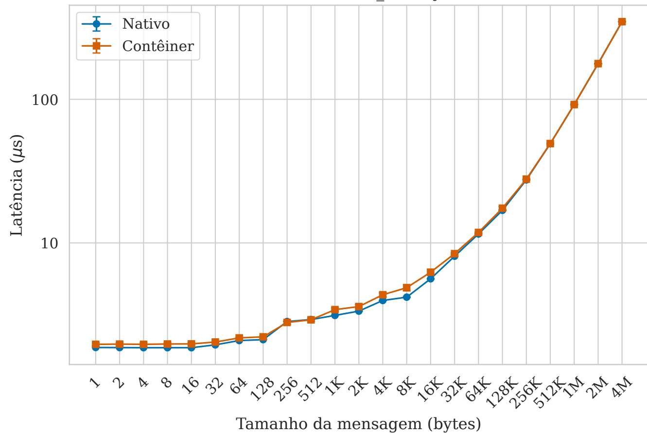
Latência (osu_latency)
