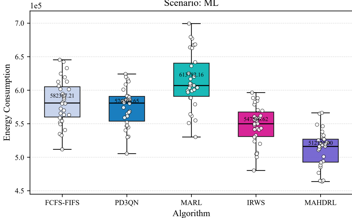
Scenario: ML
