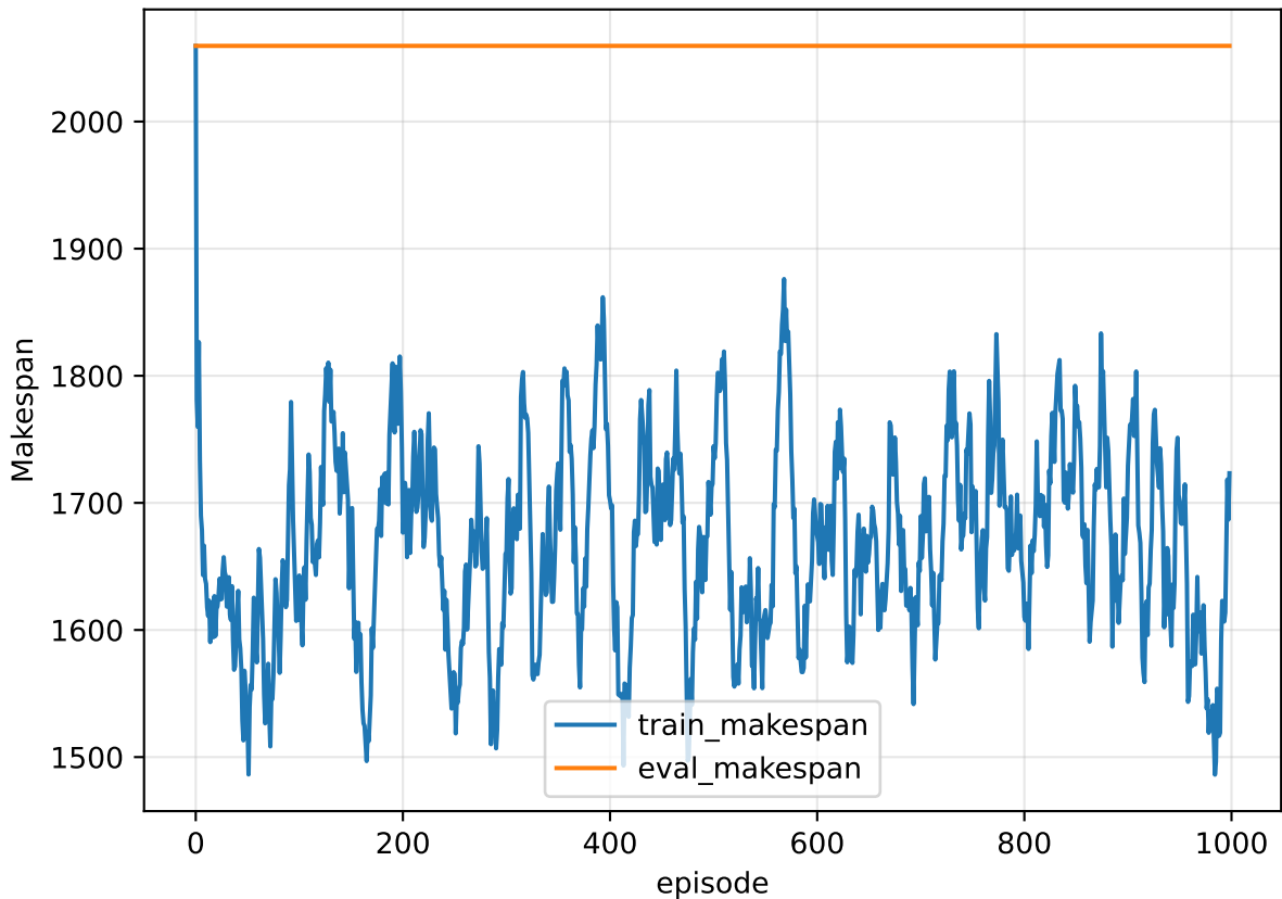
PD3QN: Makespan
