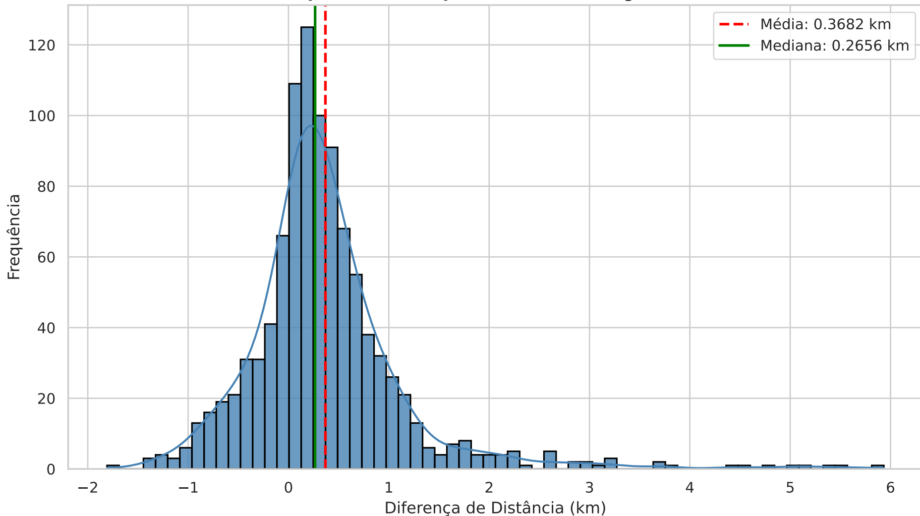
Distribuição da Diferença de Distância (Original vs Offset)
