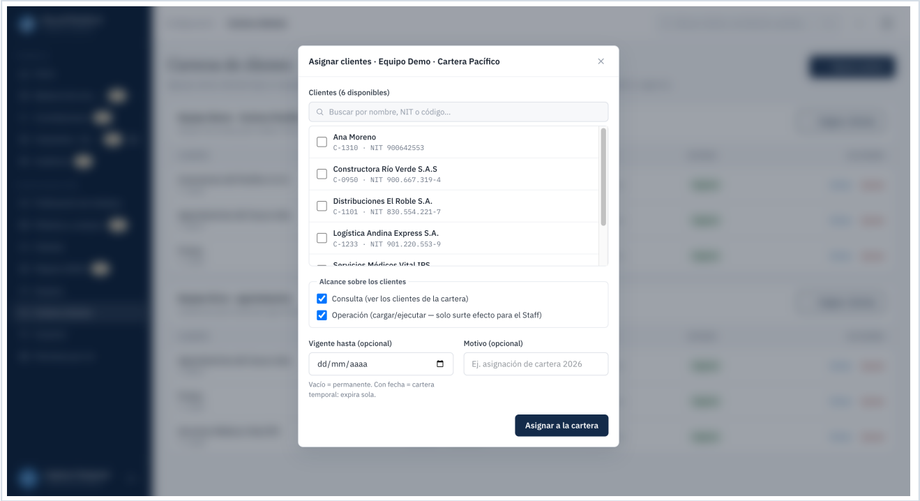
■ Modal «Asignar clientes»: se eligen uno o varios clientes y se marcan las casillas de Alcance — Consulta (lectura) y Operación (escritura, que solo surte efecto para el Staff).
