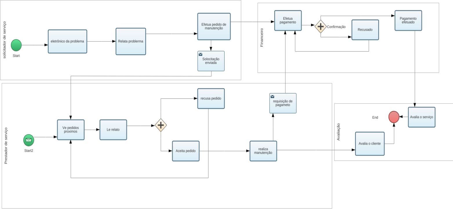
Ds2 Diagrama de atividades.
