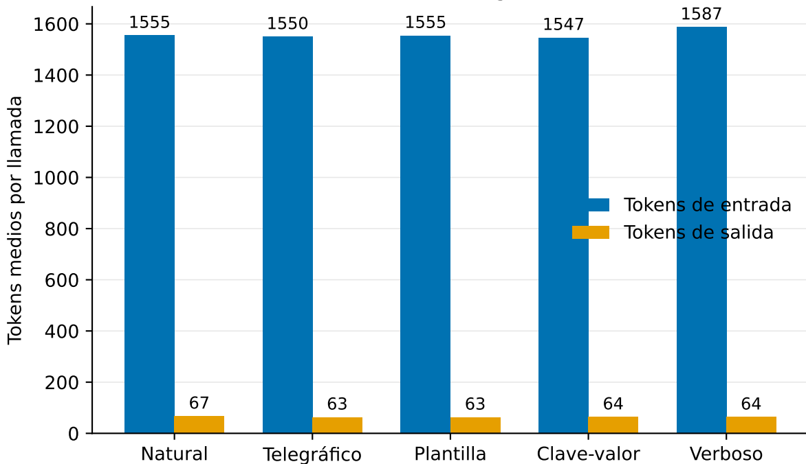
Consumo de tokens según el formato
