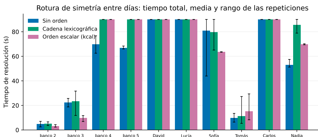
Figura 7.4: Tiempo de resolución por caso y brazo, media y rango de las 5 repeticiones. Donde las tres barras tocan el límite, la diferencia está en el estado y en la calidad del incumbente, que recogen las tablas de la sección D.3 del Anexo D.
