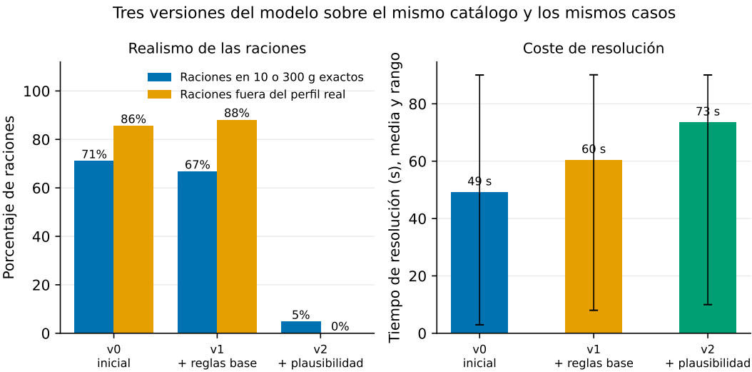
Figura 7.1: Realismo de las raciones frente a coste de resolución por versión del modelo. A la derecha, media y rango del tiempo de resolución.
