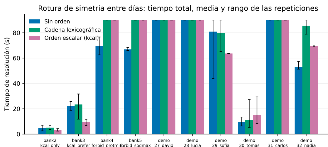
Figura 7.6: Tiempo de resolución por caso y brazo, media y rango de las 5 repeticiones. Donde las tres barras tocan el límite, la diferencia está en el estado y en la calidad del incumbente, que recoge la tabla 7.11.
