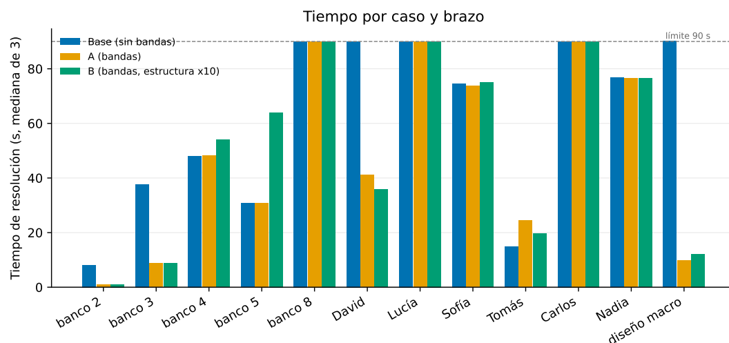
Figura D.2: Tiempo de resolución por caso y brazo (mediana de 3 repeticiones).
