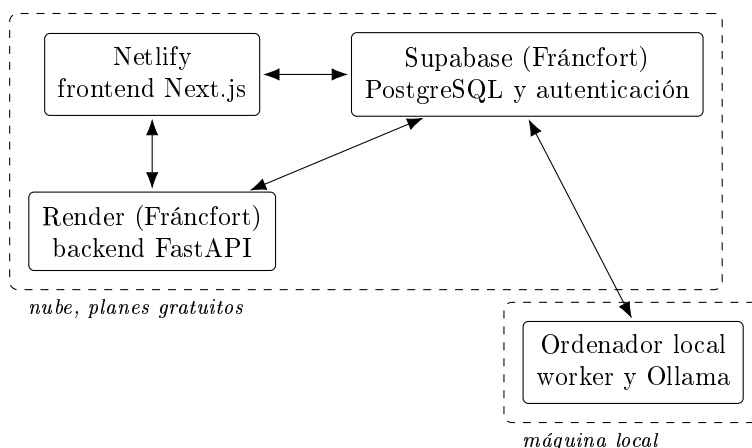
Figura 4.7: Despliegue: tres patas en planes gratuitos de nube y el worker en una máquina local, todas comunicadas a través de la base de datos o de llamadas de servidor a servidor.
