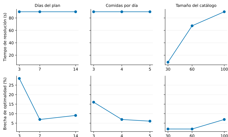
Figura 7.3: Escalado por dimensión: tiempo de resolución (arriba) y brecha de optimalidad (abajo). Con el tiempo en el límite, la brecha separa las configuraciones.
