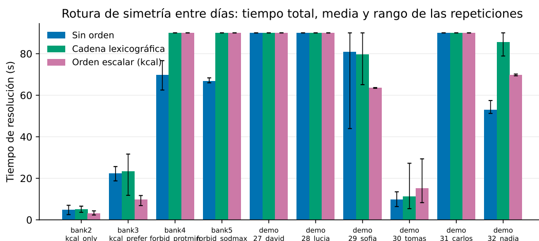
Figura 7.4: Tiempo de resolución por caso y brazo, media y rango de las 5 repeticiones. Donde las tres barras tocan el límite, la diferencia está en el estado y en la calidad del incumbente, que recogen las tablas de la sección D.3 del Anexo D.
