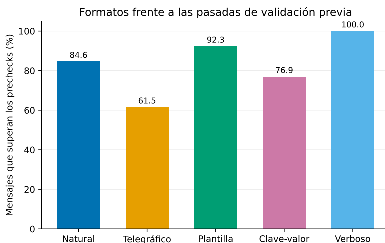
Figura 7.6: Mensajes que superan las pasadas de validación previa, por formato (una pasada por cada uno de los 65 pares formato-mensaje).
