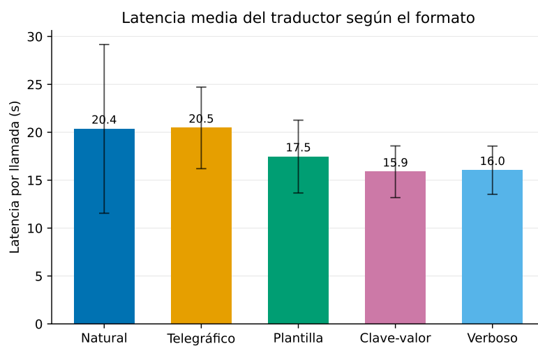
Figura D.6: Latencia por llamada al traductor, por formato.
