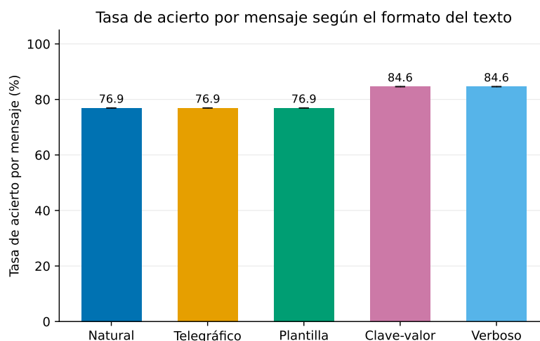
Figura D.4: Tasa de acierto por mensaje según el formato (media de 3 repeticiones, desviación cero).
