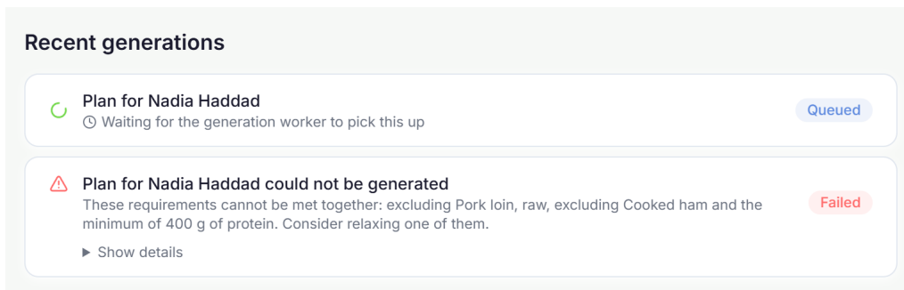
Figura 4.6: El apartado de generaciones recientes con el worker apagado: la tarea nueva queda en cola y, pasados dos minutos, la interfaz avisa de que espera al worker; debajo, una generación anterior que falló conserva su explicación.
