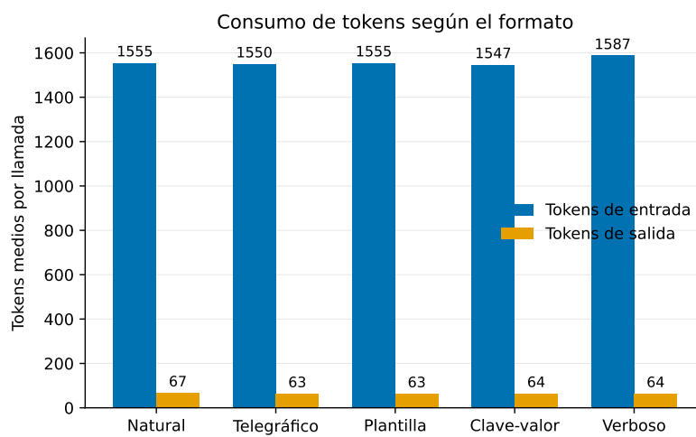
Figura D.7: Tokens de entrada y salida por llamada, por formato.
