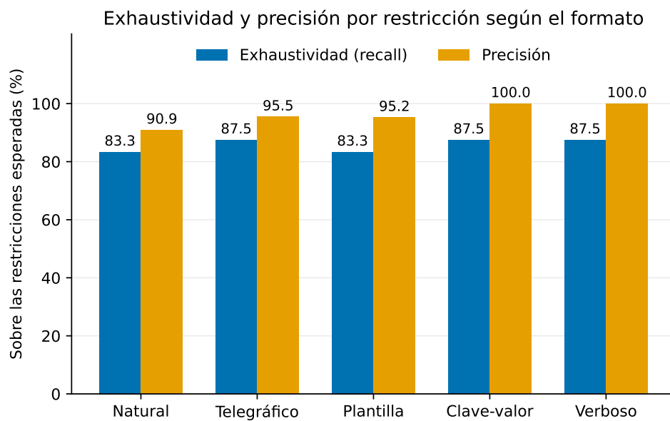
Figura D.5: Exhaustividad y precisión por restricción, por formato.
