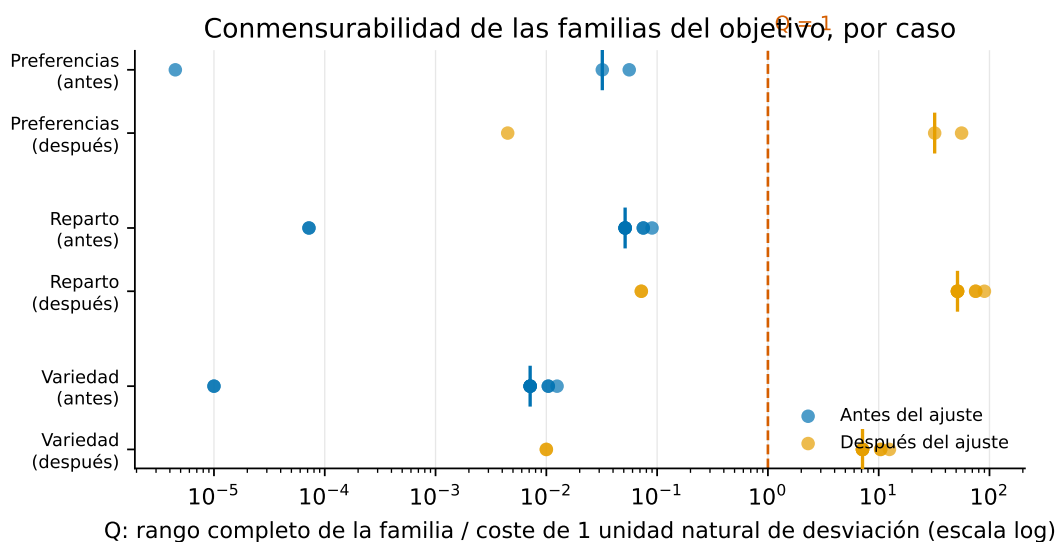
Figura D.1: Q de cada familia en cada caso, antes y después del ajuste (escala logarítmica). La línea discontinua marca Q = 1 ; la barra vertical de cada serie es su mediana.
