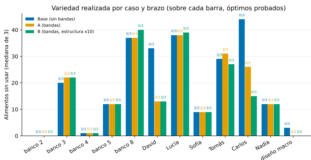
Figura 7.2: Bandas de tolerancia: alimentos del catálogo sin usar por caso y brazo (base sin bandas, A con bandas, B con bandas y estructura por diez), con los óptimos probados de tres repeticiones sobre cada barra. Los tiempos y las tablas por caso están en la sección D.4 del Anexo D.
