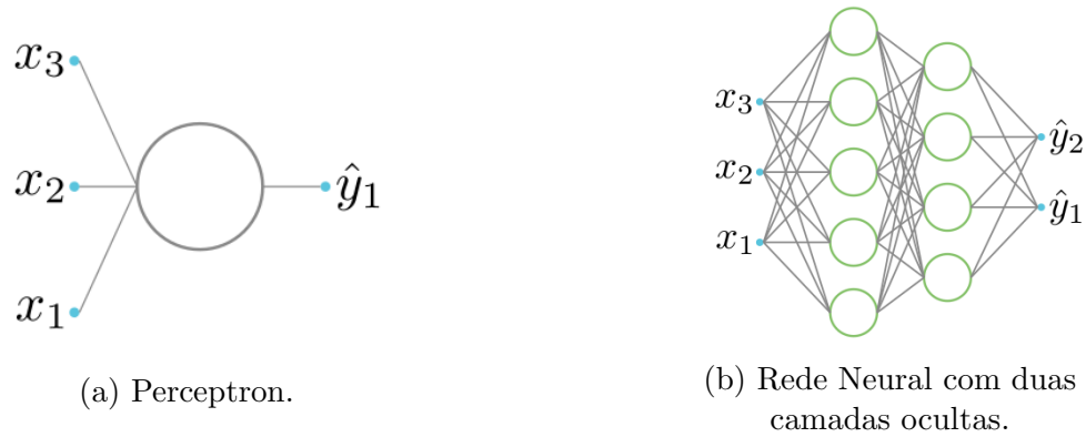
Figura 1.5: Estrutura básica de uma unidade e uma rede neural com duas camadas ocultas.
