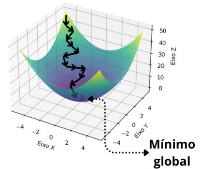
(c) Gradiente Descendente Estocástico (SGD).
