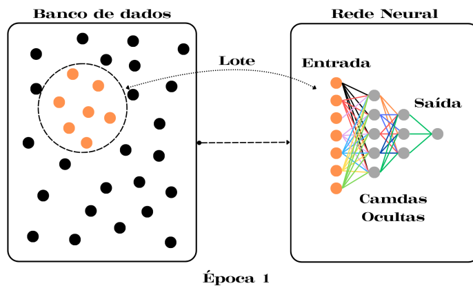
(a) Separando em Lotes o banco de dados para o SGD.
