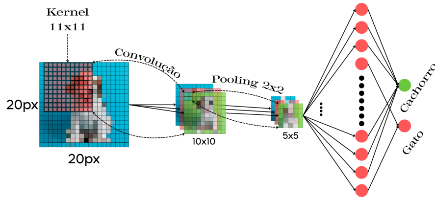
Figura 1.19: Arquitetura típica de uma Rede Neural Convolucional com uma camada de convolução e uma camada de pooling, em que é enviado para rede a imagem de um cachorro e é feita a classificação do objeto na imagem.
