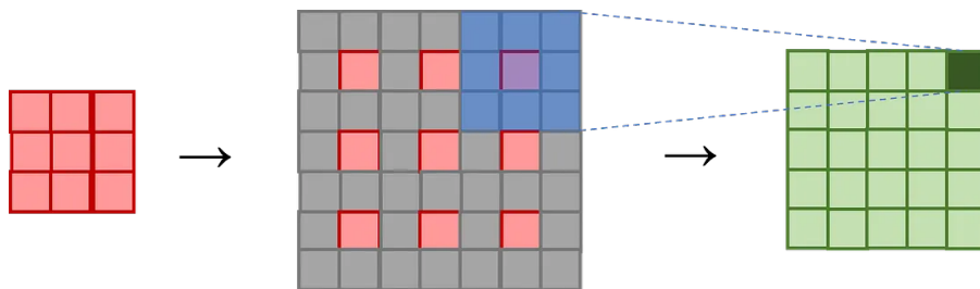
Figura 1.18: Convolução transposta. Uma convolução de kernel 3 \times 3 com stride 1 em uma imagem 5 \times 5 geraria uma imagem de dimensões 3 \times 3 . A convolução transposta aplicada na imagem 3 \times 3 (vermelha) para se obter uma imagem 5 \times 5 (verde) é feita em duas etapas.
