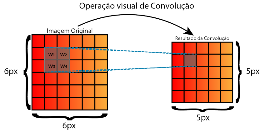
Figura 1.14: Exemplo de convolução bidimensional. A função X(t) é convoluída com o kernel W(a) para produzir a saída S(t) .
