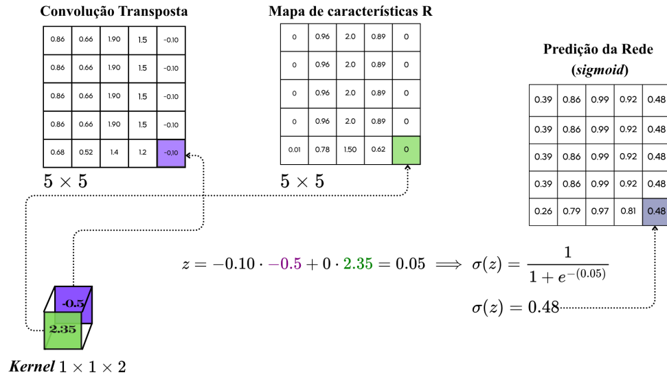
Figura 3.11: Aplicação da última camada de convolução para gerar a imagem de saída Y .
