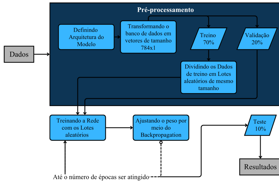
Figura 1.15: Fluxo de dados durante o processo de treinamento e avaliação da rede neural.
