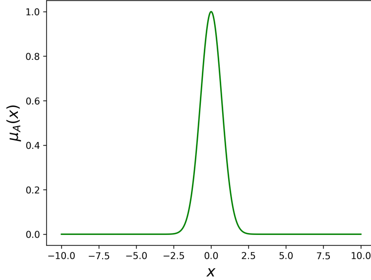
Figura 3.15: Função de pertinência gaussiana.
