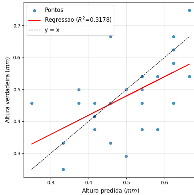
Figura 4.15: Reta de regressão linear e R^2 entre as medidas preditas e as medidas reais da EGG para o modelo de U-Net Fuzzy.
