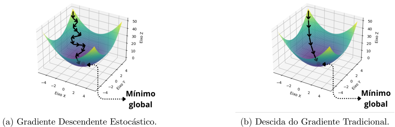
Figura 1.7: Comparação entre os métodos de descida do gradiente.
