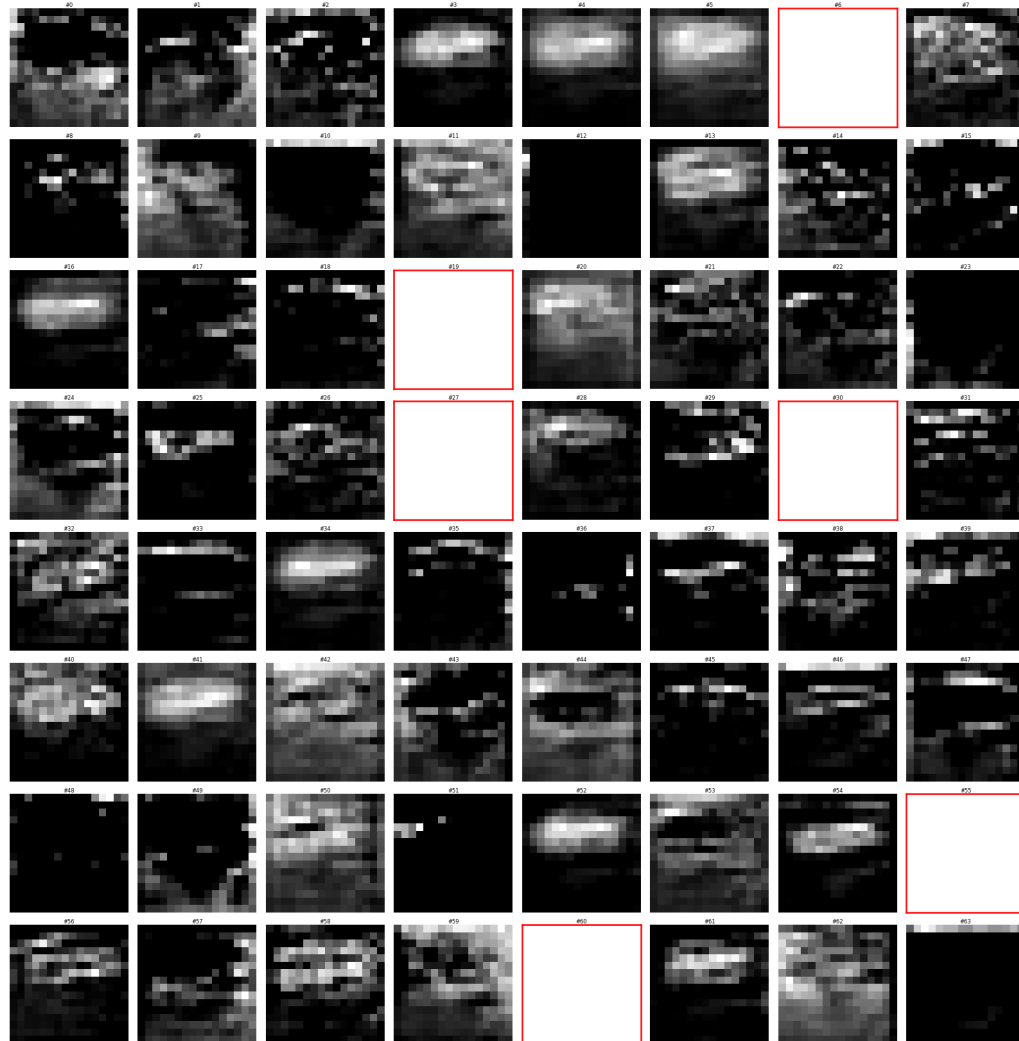
Figura 4.18: Mapa de características na última etapa de convolução do encoder da U-Net.
