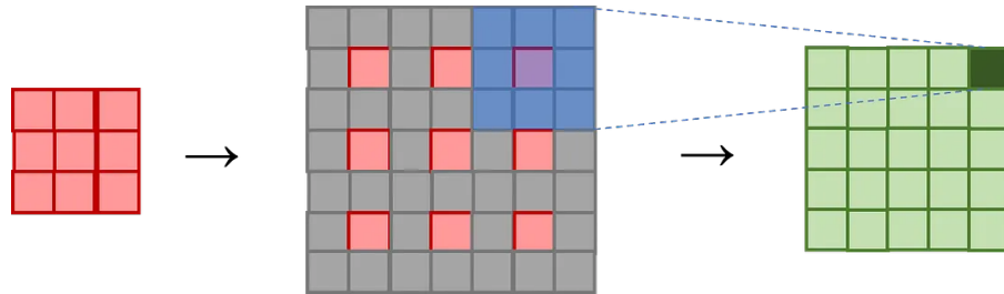
Figura 1.18: Convolução transposta. Uma convolução de kernel 3 \times 3 com stride 1 em uma imagem 5 \times 5 geraria uma imagem de dimensões 3 \times 3 . A convolução transposta aplicada na imagem 3 \times 3 (vermelha) para se obter uma imagem 5 \times 5 (verde) é feita em duas etapas.
