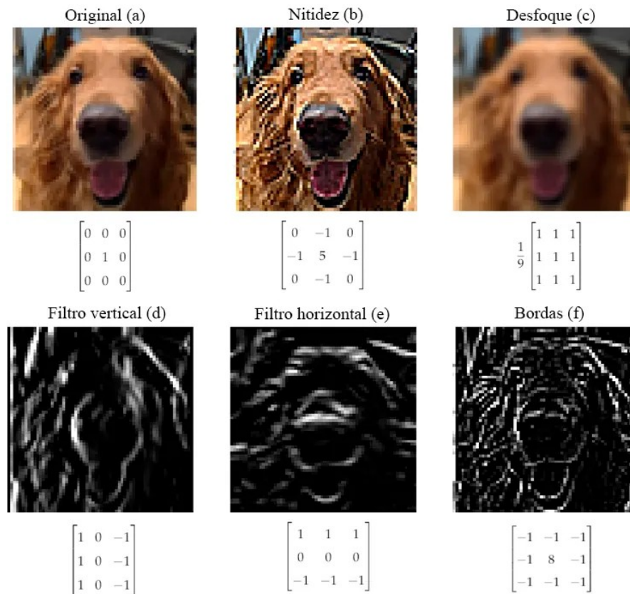
Figura 1.15: Aplicações de diferentes kernels em uma imagem. A imagem original é representada em (a), juntamente com o kernel identidade, que não faz modificações. Em (b) a imagem passou por um kernel que aumenta a nitidez reforçando o pixel central e aumentando a diferença dele em relação à sua vizinhança. Em (c) foi usado um kernel de desfoque, que substitui um pixel pela média dele com seus vizinhos. A imagem em (d) é o resultado de aplicar na imagem em escala de cinza um kernel que reforça suas linhas verticais, enquanto (e) reforça suas linhas horizontais. O kernel em (f) reforça os contornos (bordas) da imagem.
