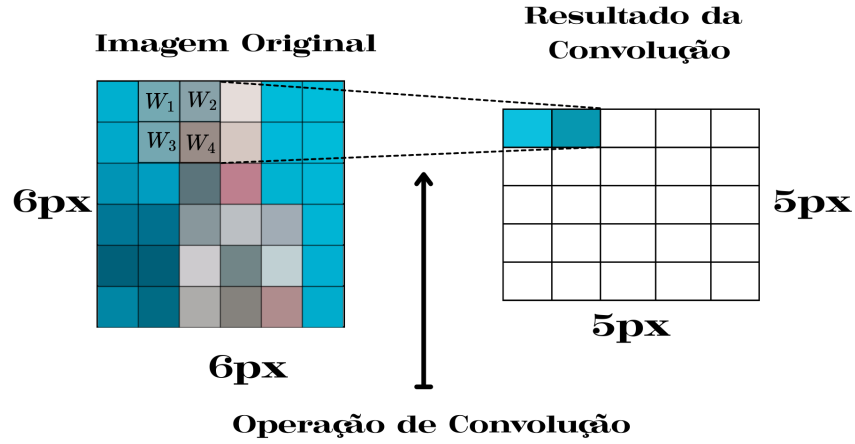
Figura 1.14: Exemplo de convolução bidimensional. A função X(t) é convoluída com o kernel W(a) para produzir a saída S(t) .
