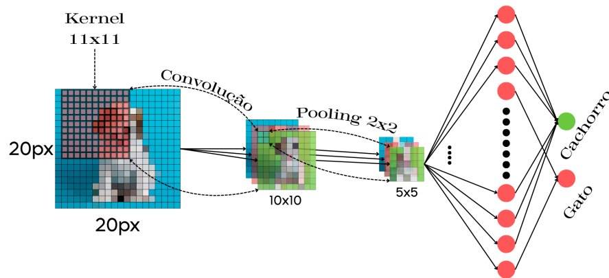
Figura 1.19: Arquitetura típica de uma Rede Neural Convolutacional com uma camada de convolução e uma camada de pooling, em que é enviado para rede a imagem de um cachorro e é feita a classificação do objeto na imagem.
