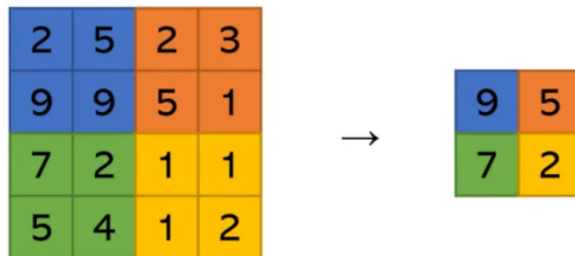
Figura 1.17: Exemplo de Max Pooling com tamanho de 2x2. A imagem original é reduzida para a imagem menor após a aplicação do Max Pooling. Cada bloco de 2x2 pixels na imagem original é substituído pelo valor máximo dentro desse bloco na imagem reduzida.
