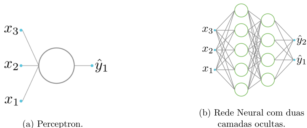
Figura 1.5: Estrutura básica de uma unidade e uma rede neural com duas camadas ocultas.
