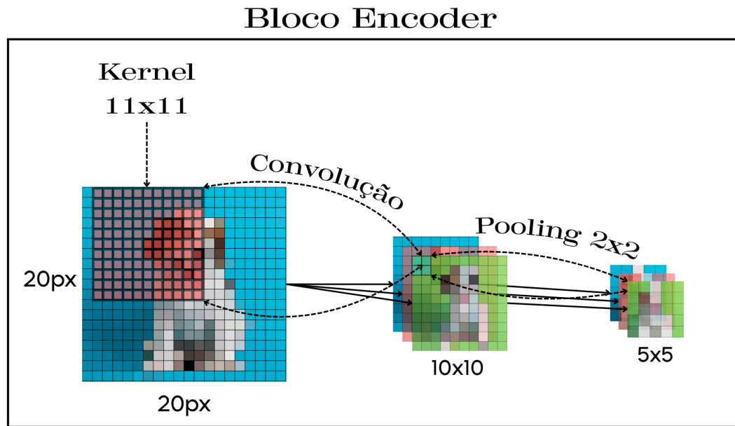
(a) Encoder da U-Net, onde as setas indicam as operações de convolução e pooling que extraem características da imagem de entrada.
