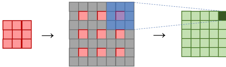
Figura 1.18: Convolução transposta. Uma convolução de kernel 3x3 com stride 1 em uma imagem 5 \times 5 geraria uma imagem de dimensões 3 \times 3 . A convolução transposta aplicada na imagem 3 \times 3 (vermelha) para se obter uma imagem 5 \times 5 (verde) é feita em duas etapas.
