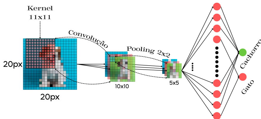
Figura 1.19: Arquitetura típica de uma Rede Neural Convolutiva com uma camada de convolução e uma camada de pooling, em que é enviado para rede a imagem de um cachorro e é feita a classificação do objeto na imagem.
