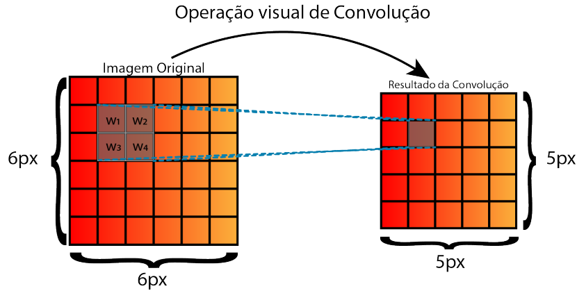
Figura 1.13: Exemplo de convolução bidimensional. A função X(t) é convoluída com o kernel W(a) para produzir a saída S(t) .
