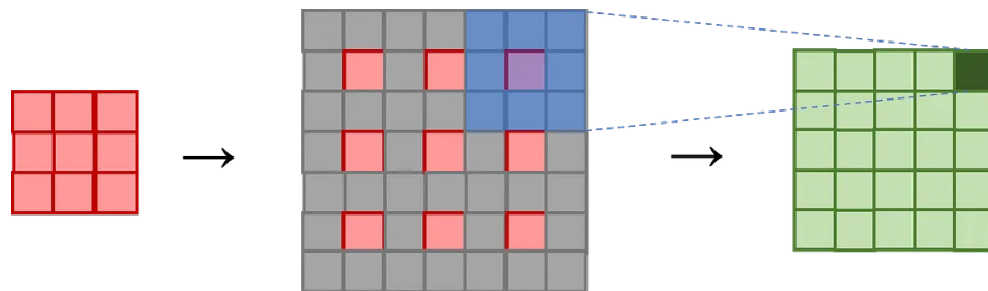
Figura 1.17: Convolução transposta. Uma convolução de kernel 3 \times 3 com stride 1 em uma imagem 5 \times 5 geraria uma imagem de dimensões 3 \times 3 . A convolução transposta aplicada na imagem 3 \times 3 (vermelha) para se obter uma imagem 5 \times 5 (verde) é feita em duas etapas. Primeiramente (centro) se insere pixels de valor 0, representados pela cor cinza, entre os pixels da imagem original, juntamente com pixels de borda. Em seguida se faz uma convolução nessa imagem alterada também usando um kernel 3 \times 3 e stride 1.
