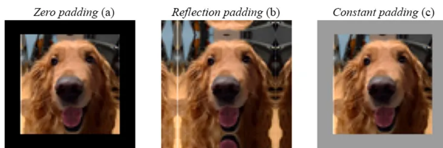
Figura 1.15: Aplicação de padding em uma imagem. Em (a) a imagem original passou por zero padding. Em (b) a imagem original passou por reflection padding . A imagem em (c) passou por um padding constante, semelhante em (a), mas com valor diferente de zero.
