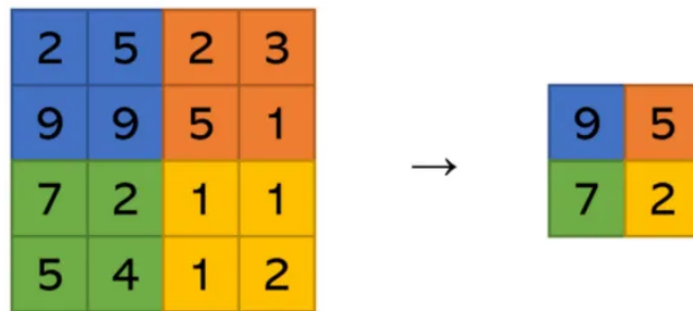
Figura 1.16: Exemplo de Max Pooling com tamanho de 2x2. A imagem original é reduzida para a imagem menor após a aplicação do Max Pooling. Cada bloco de 2x2 pixels na imagem original é substituído pelo valor máximo dentro desse bloco na imagem reduzida.
