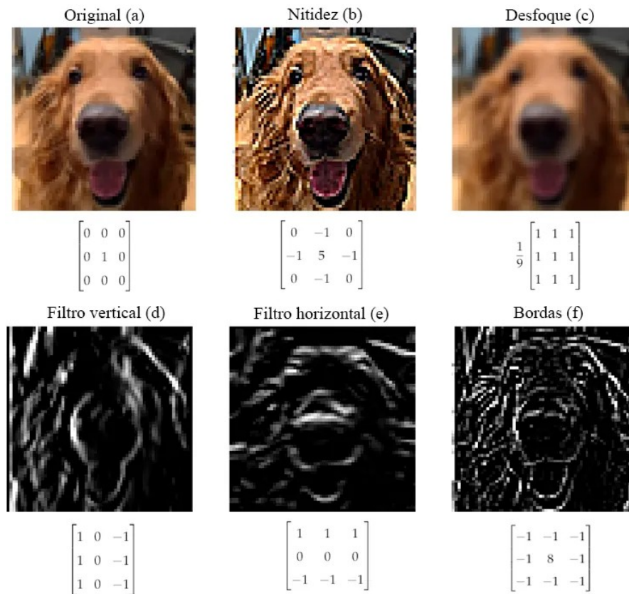
Figura 1.14: Aplicações de diferentes kernels em uma imagem. A imagem original é representada em (a), juntamente com o kernel identidade, que não faz modificações. Em (b) a imagem passou por um kernel que aumenta a nitidez reforçando o pixel central e aumentando a diferença dele em relação à sua vizinhança. Em (c) foi usado um kernel de desfoque, que substitui um pixel pela média dele com seus vizinhos. A imagem em (d) é o resultado de aplicar na imagem em escala de cinza um kernel que reforça suas linhas verticais, enquanto (e) reforça suas linhas horizontais. O kernel em (f) reforça os contornos (bordas) da imagem.
