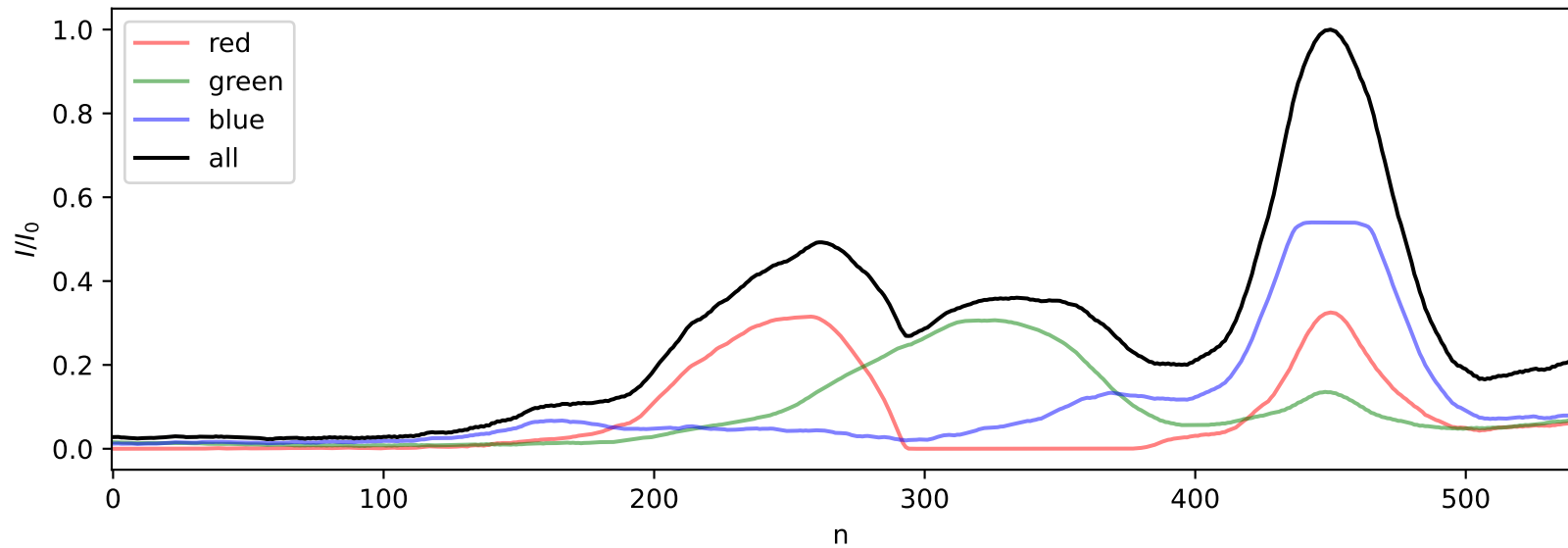
Зависимость относительной интенсивности столбца кадра от номера столбца
