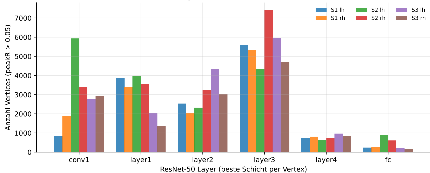
Verteilung der besten Schicht (RSA, k50)
