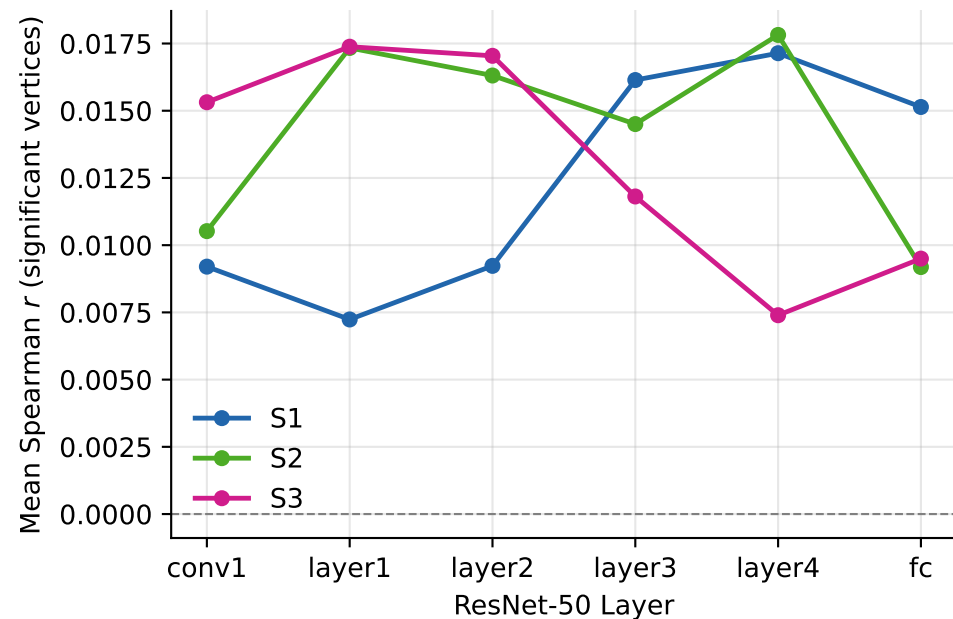
RSA (Spearman r ) per Layer
