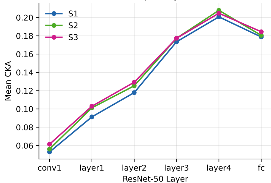
CKA per Layer
