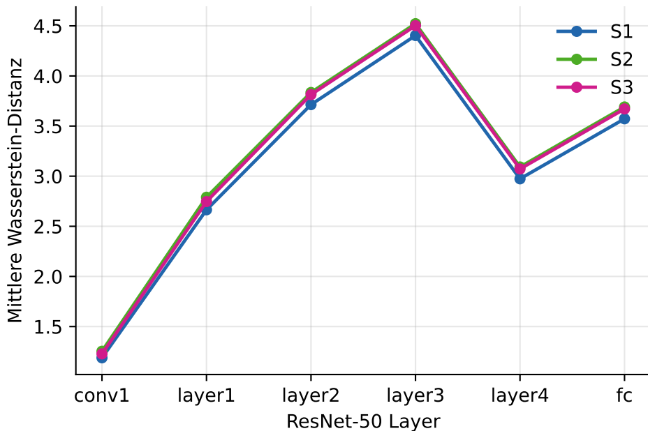
TDA Wasserstein-Distanz H_1 per Layer
