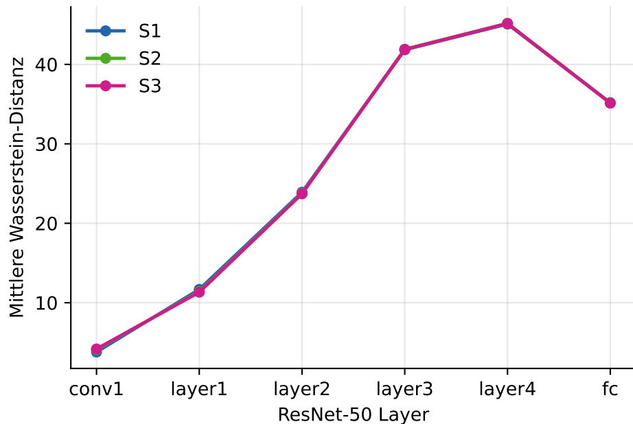
TDA Wasserstein-Distanz H_0 per Layer
