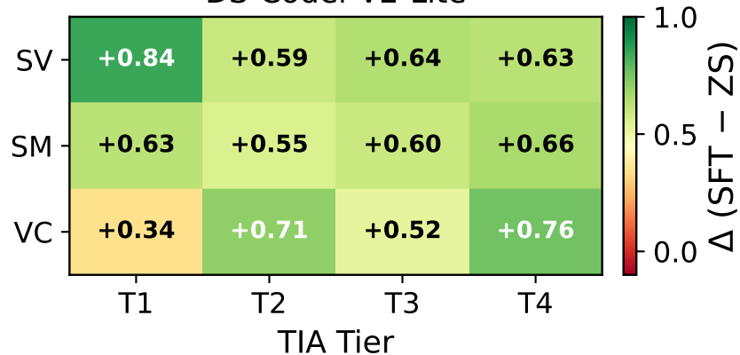
DS-Coder-V2-Lite
