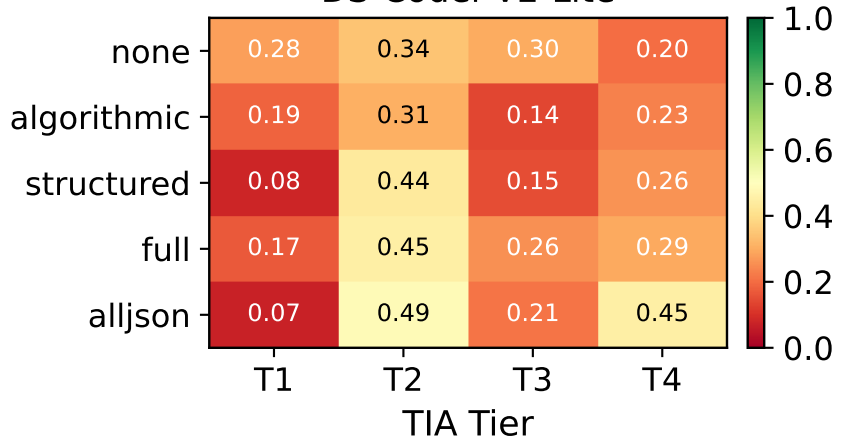
DS-Coder-V2-Lite
