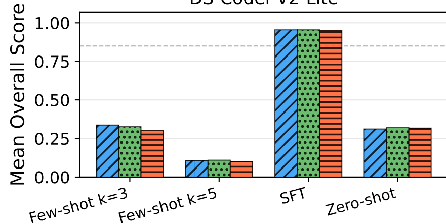
DS-Coder-V2-Lite
