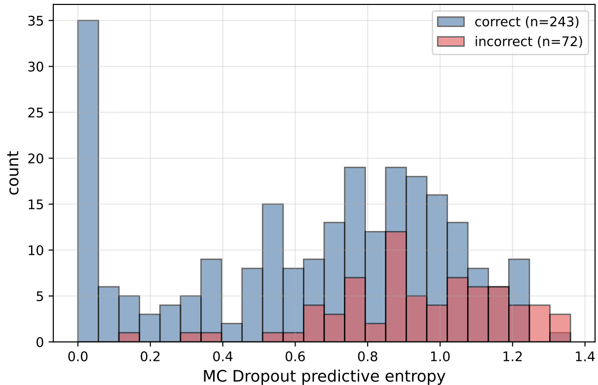
VGG16
