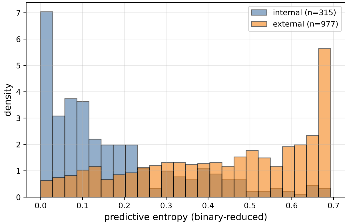
VGG16
