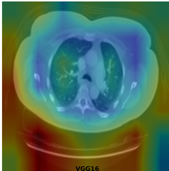
VGG16
