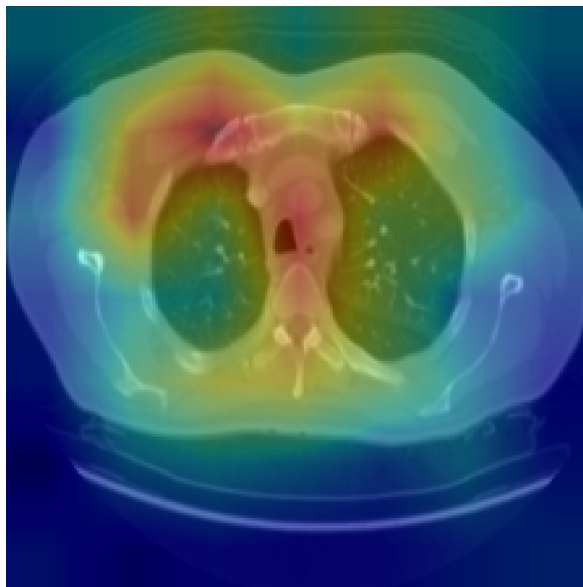
VGG16
