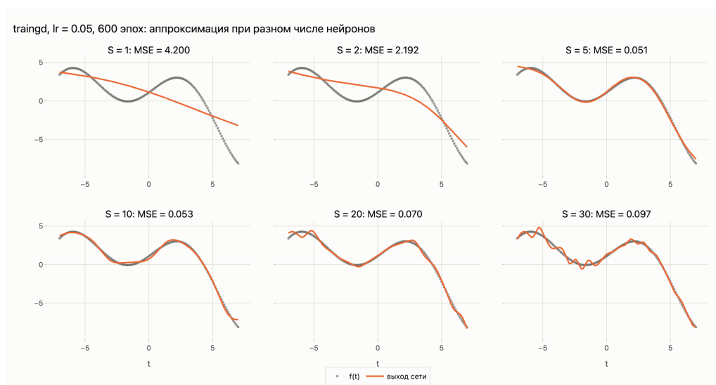
Рисунок Л3.1 – Аппроксимация при разном числе нейронов (градиентный спуск, \eta = 0,05 , 600 эпох)
