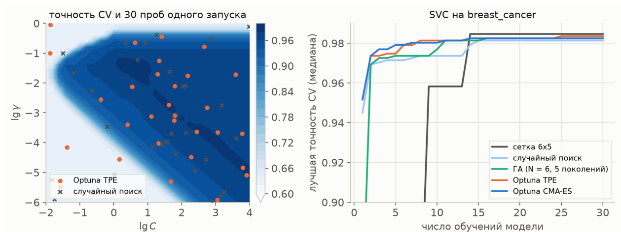
Рисунок Л8.2 – Слева — точность кросс-валидации на плоскости гиперпараметров и 30 проб TPE и случайного поиска в одном запуске; справа — медиана лучшей найденной точности
