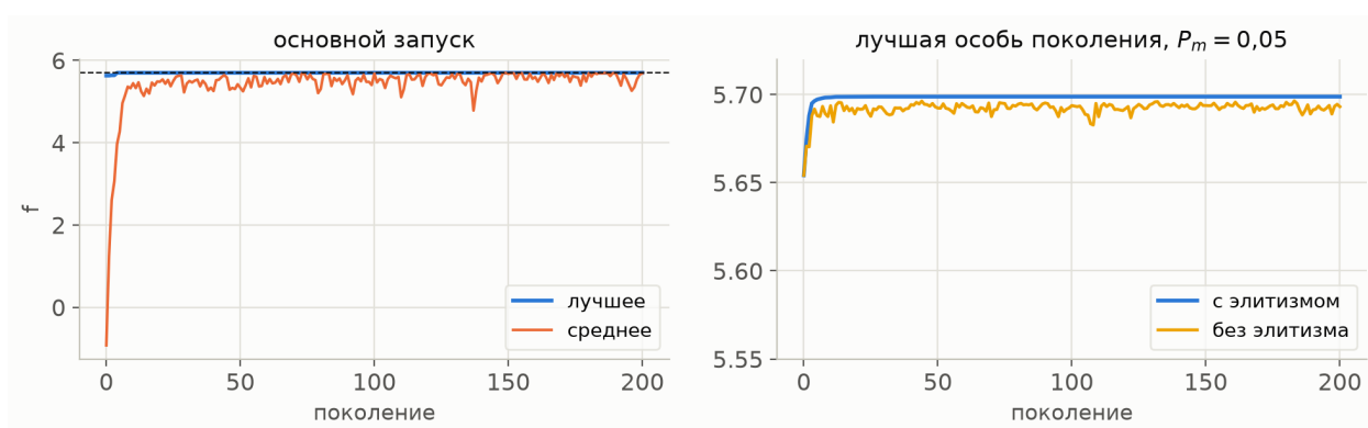
Рисунок Л5.2 – Слева — лучшее и среднее значения функции в основном запуске (пунктир — f^* ); справа — лучшая особь поколения с элитизмом и без него (среднее по 30 запускам, P_m = 0,05 )
