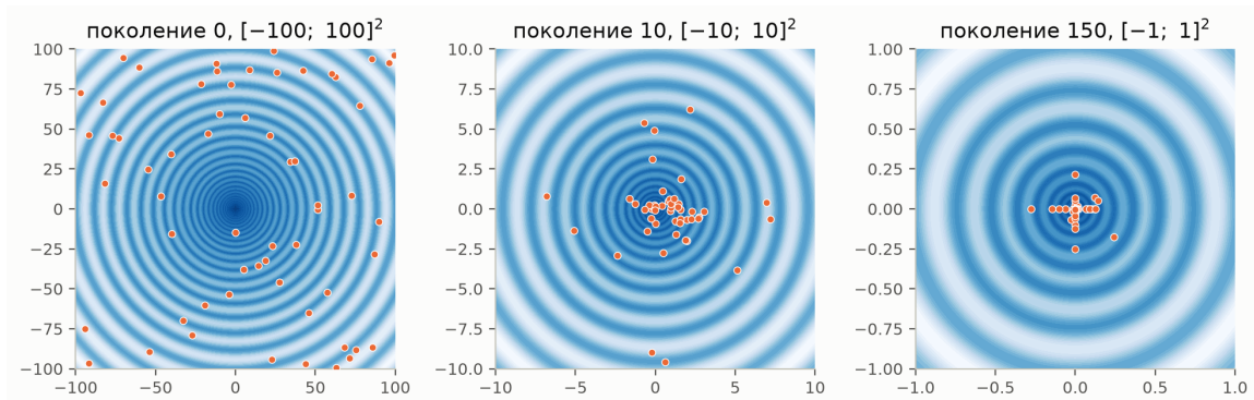
Рисунок Л6.3 – Популяция вещественного ГА на линиях уровня функции Шаффера F7 (масштаб осей уменьшается)
