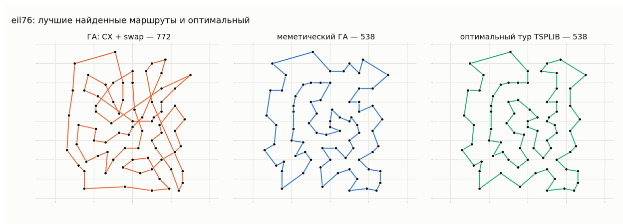
Рисунок Л7.1 – Лучшие найденные маршруты и опубликованный оптимальный тур eil76
