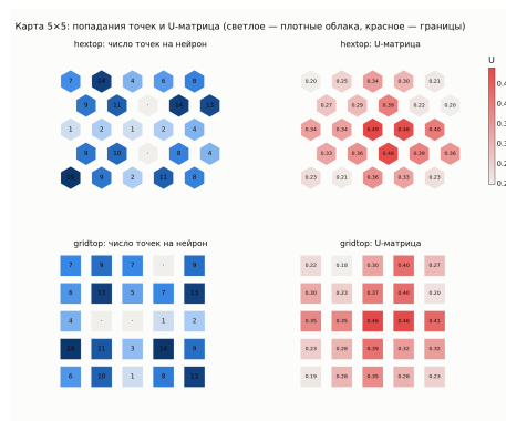
Рисунок Л4.2 – Карта 5 \times 5 : число попаданий точек на нейрон и U-матрица
