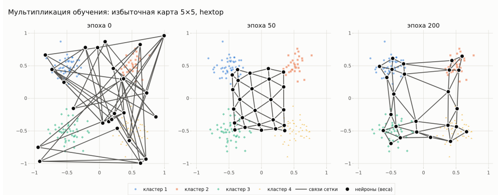
Рисунок Л4.1 – Мультипликация обучения избыточной карты 5 \times 5 hextop: эпохи 0, 50 и 200
