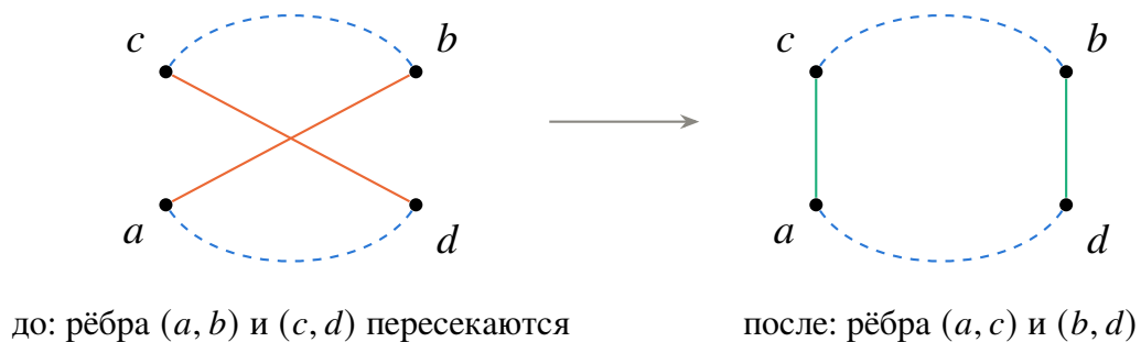
Рисунок 7.2 – Ход 2-орт: рёбра (a, b) , (c, d) заменяются на (a, c) , (b, d) , и путь от b до c проходится в обратном направлении (пунктир — остальная часть тура)
