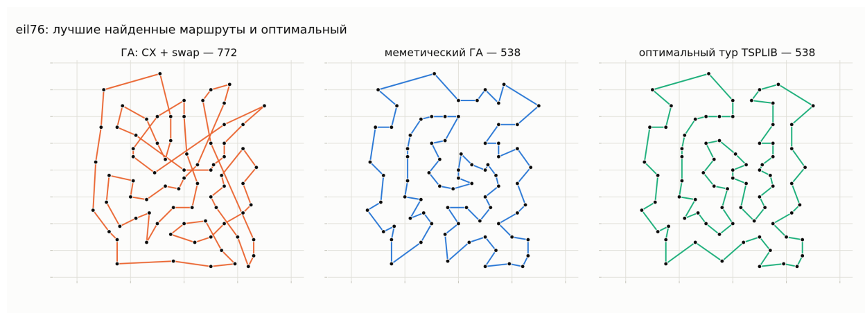
Рисунок Л7.2 – Лучшие найденные маршруты и опубликованный оптимальный тур eil76
