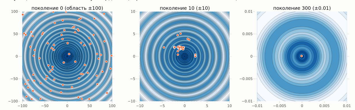
Рисунок Лб.2 – Популяция ГА на линиях уровня функции Шаффера F7: поколения 0, 10 и 300 (масштаб осей уменьшается)
