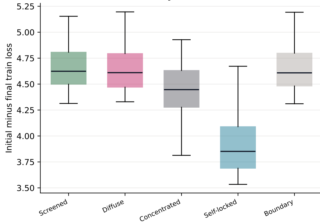
TinyStories
