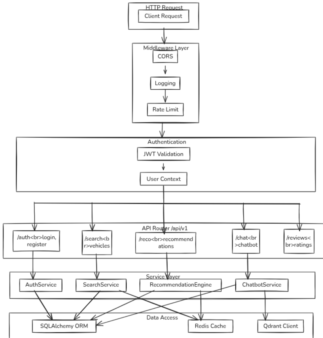
Hình 4.3: Kiến trúc phân tầng của Backend API
